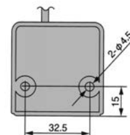
取付参考寸法
