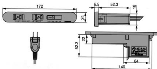
共通寸法
