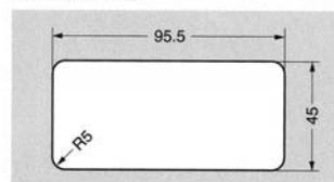
【取付穴加工図】
