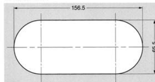
【取付穴加工図】
