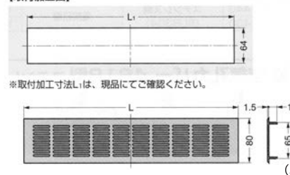
【取付加工図】
