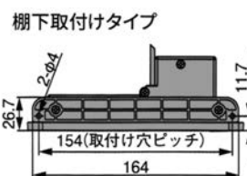
取付参考寸法
