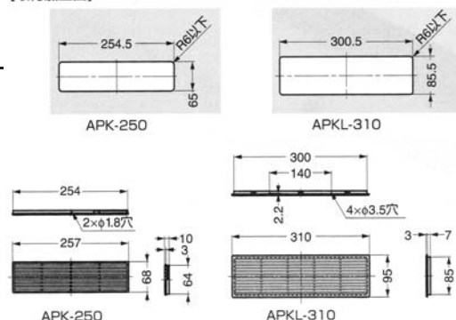
【取付加工図】
