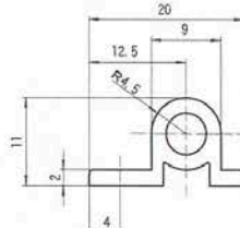
アルミ断面図
